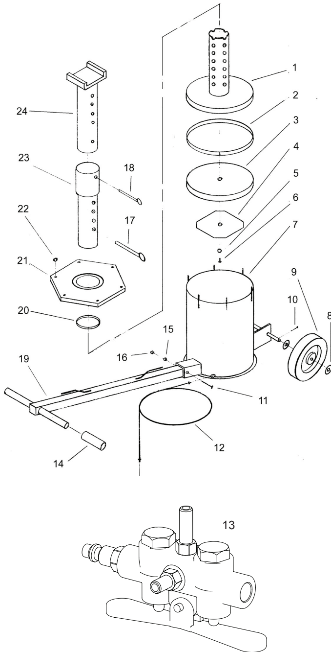
Figure 4 : Illustration des pièces de rechange du modèle 34100
