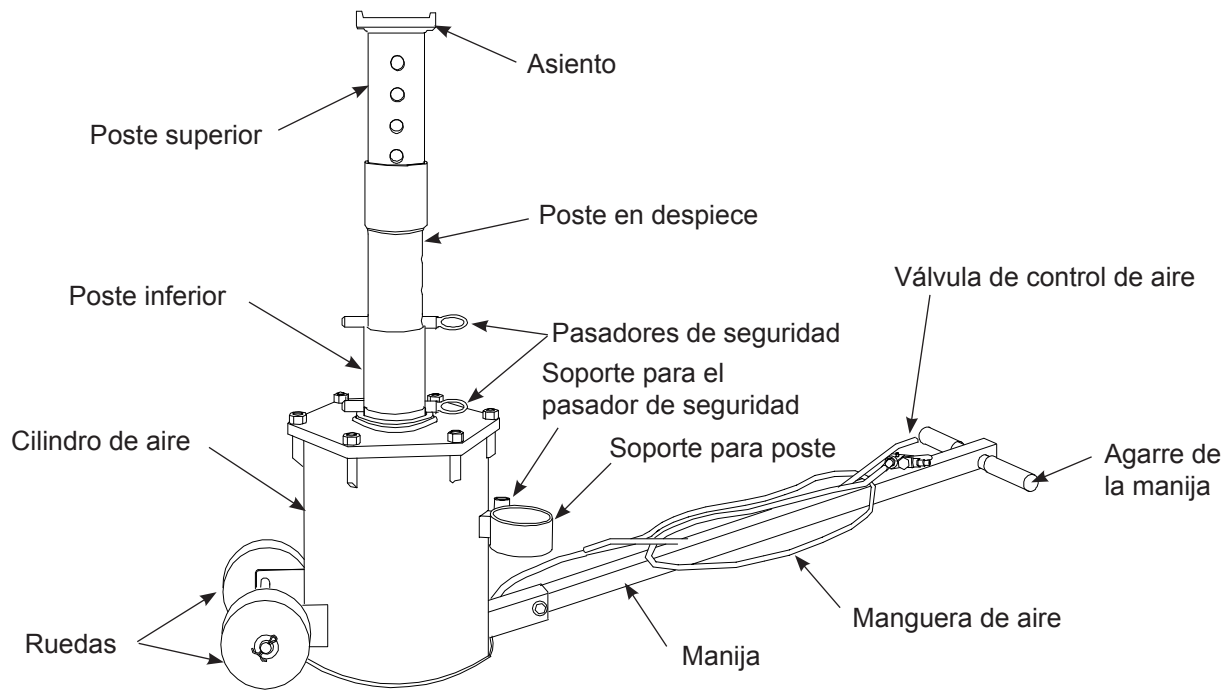
Figura 1: Componentes de un/gato neumático
