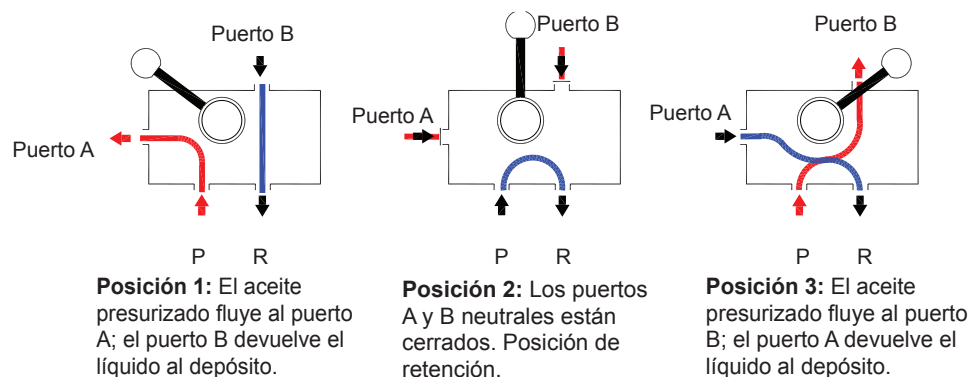
Figura 4 : Trayecto de flujo de las posiciones y operaciones de la válvula para el modelo P8701.
