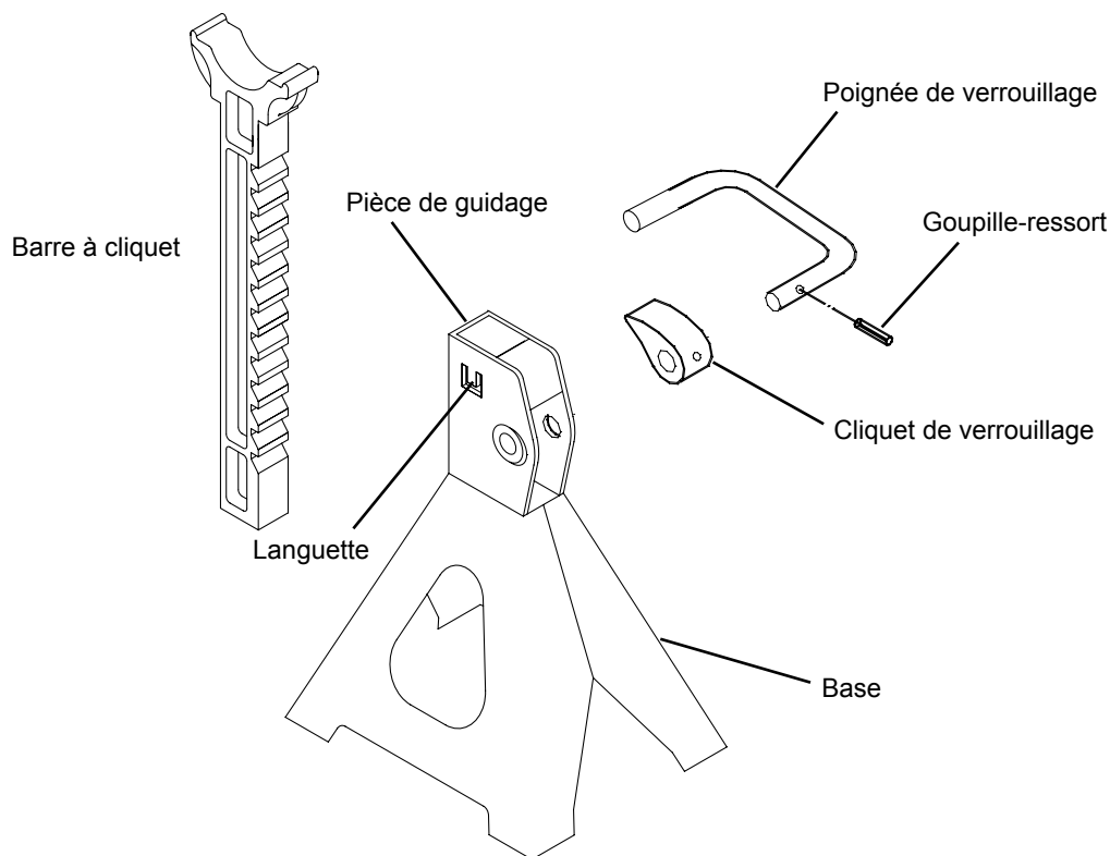
Figure 1 : Composants des béquilles de cric
